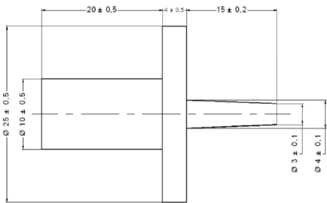
Figura 4. Probeta de prueba
