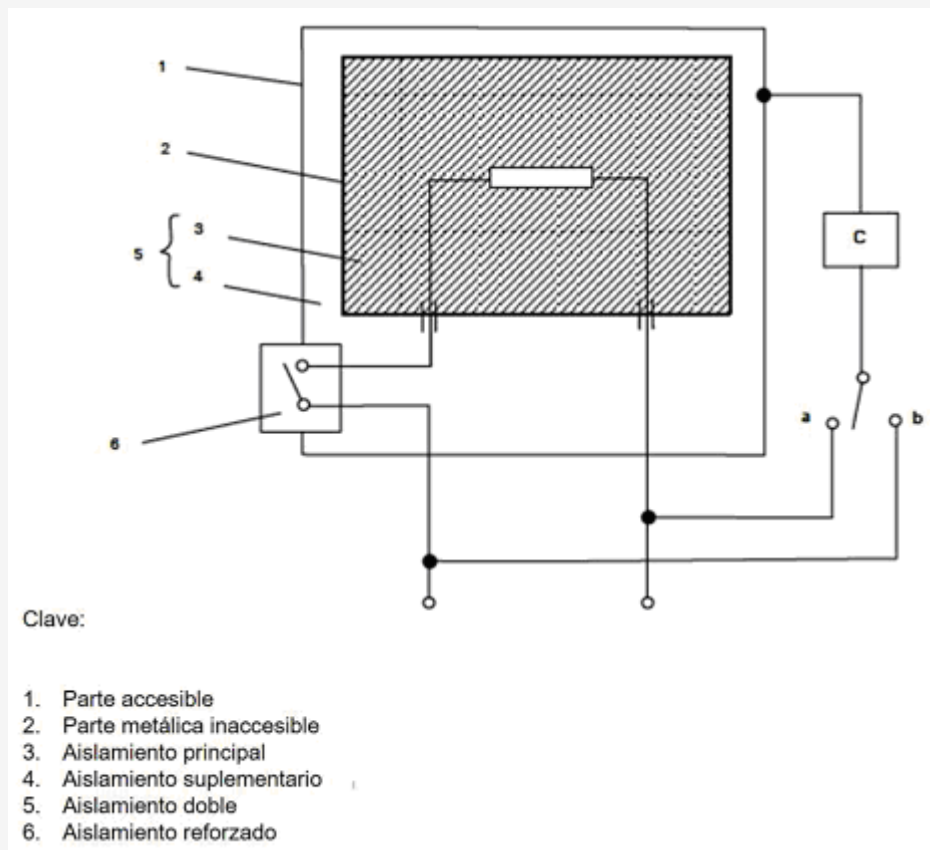
Figura 6. Aparatos distintos de Clase II monofásicos
