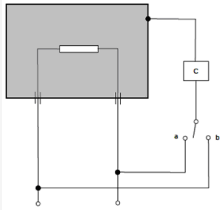
Figura 7. Aparatos de Clase II trifásicos
