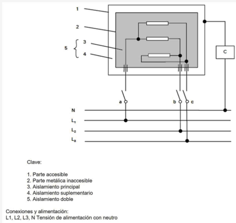
Figura 8. Diagrama para la medición de la corriente de fuga a la temperatura de operación de aparatos distintos de Clase II trifásicos
